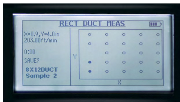
Integrierte Kanalmessanwendung (Kanaltraverse)
